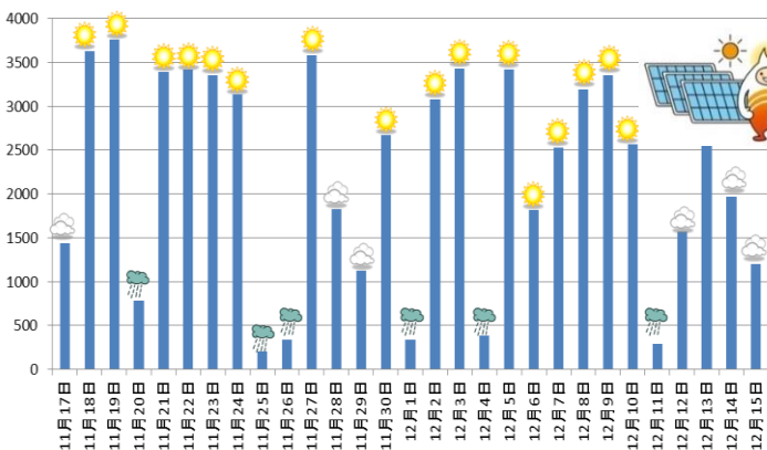
へきなんパーク11/12月 日別発電量[kWh]
