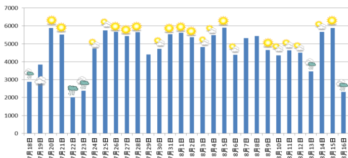
へきなんパーク7月/8月 日別発電量[kWh]
