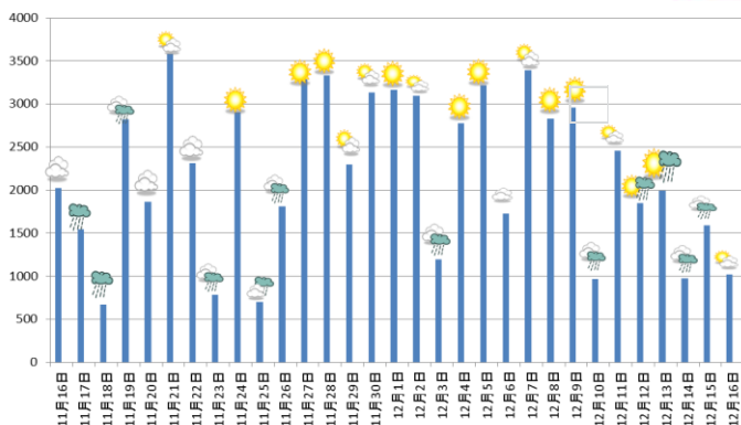
へきなんパーク11月/12月 日別発電量[kWh]
