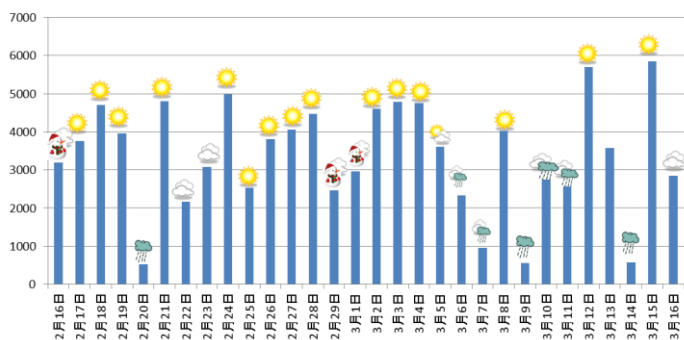
へきなんパーク2月/3月 日別発電量[kWh]
